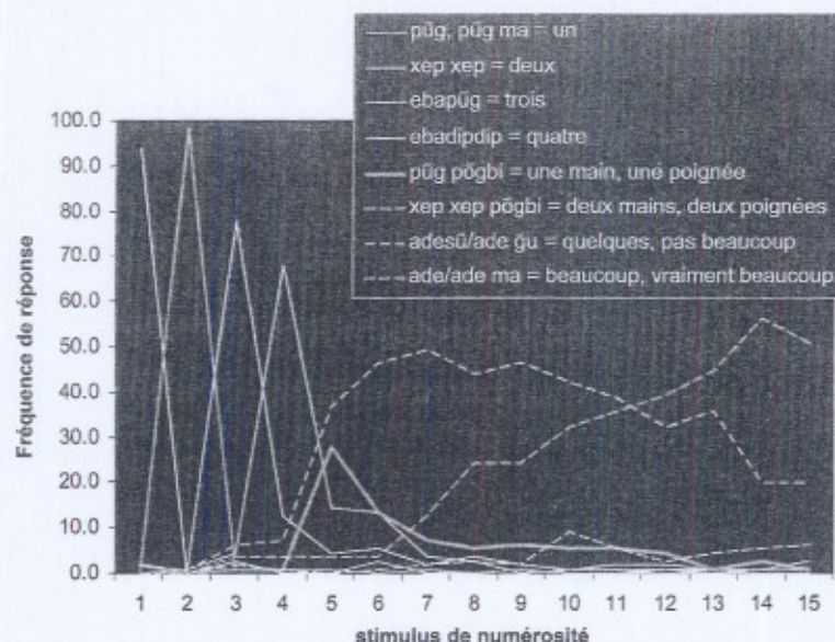
Figure 2. Dénomination de numérosité. Le lexique des nombres en mundurucú. On présentait aux participants des tableaux de 1 à 15 points, dans un ordre aléatoire, et on leur demandait de dire combien de points il y avait. Pour chaque quantité sur l'axe des x, le graphique montre la fraction des fois où elle était désignée par un mot ou une expression donnée. Nous ne présentons que les données pour les mots et locutions produits dans plus de 2,5 % de tous les essais. Pour les nombres au-delà de 5, la somme des fréquences est inférieure à 100 % : cela provient du fait que beaucoup de participants ont produit des locutions ou des phrases rares ou idiosyncratiques comme « tous mes orteils » (une liste lexicographique complète est disponible auprès des auteurs).
